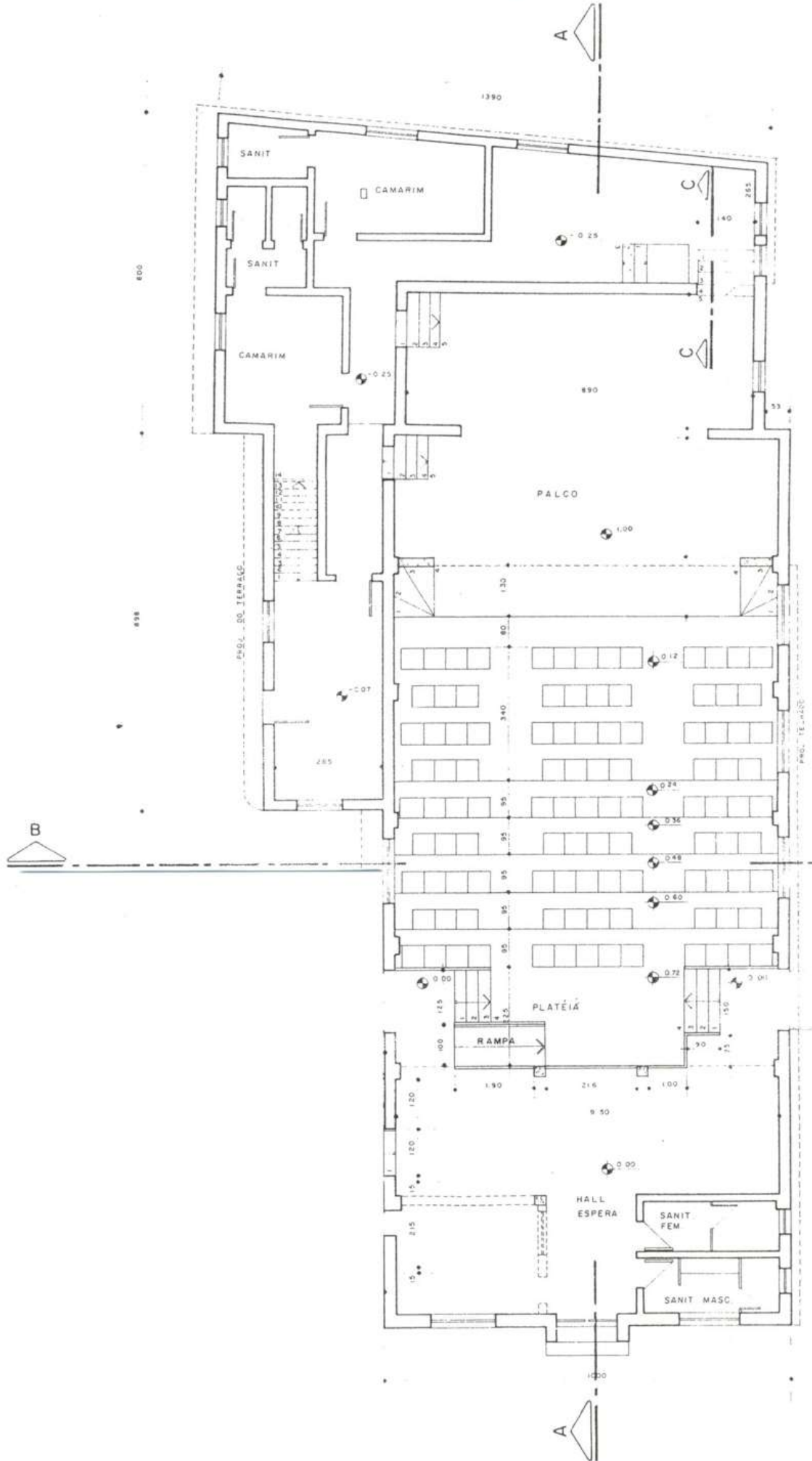
PLANTA BAIXA — PAVTO. TÉRREO ESC. 1:75
